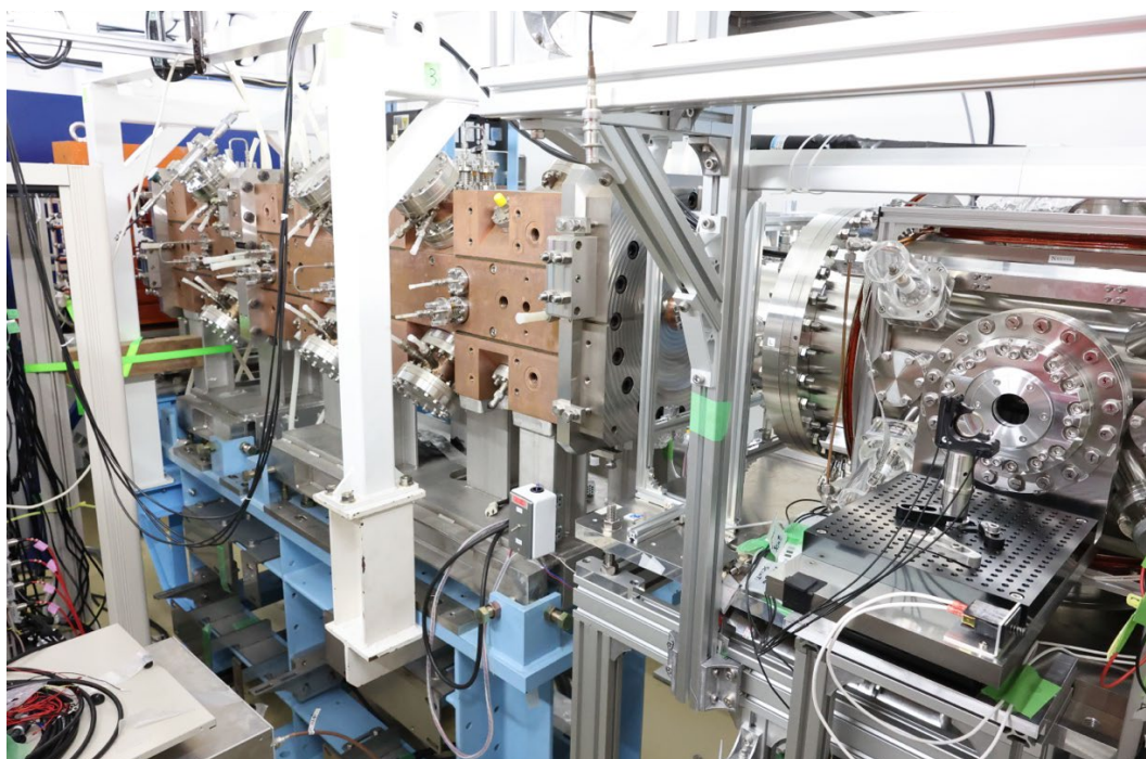
写真1 J-PARC 物質・生命科学実験施設 (MLF) ミュオン実験施設で行われたミュオン冷却・加速の実験装置。正ミュオンビームが右側から入射し、写真右手前の装置で冷却され、その左側にある高周波加速空洞で加速される。加速空洞の左奥に加速されたビームの診断装置が設置されている。
